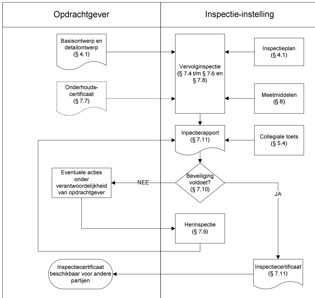
Figuur 2: Processchema vervolgininspectie
